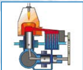
Схема Стирлинга. Красным цветом окрашена нагреваемая область, синим – охлаждаемая.
